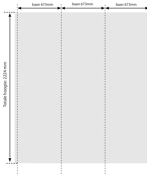
Magneetwand Expolinc 3x3 rond: Totale breedte zonder overfill = 2019mm
